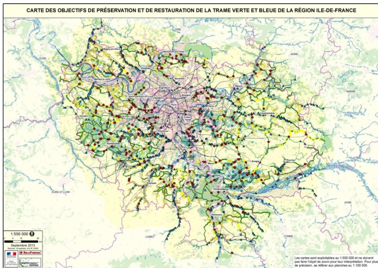
Figure 2 : Trame verte et bleue d'Île de France
