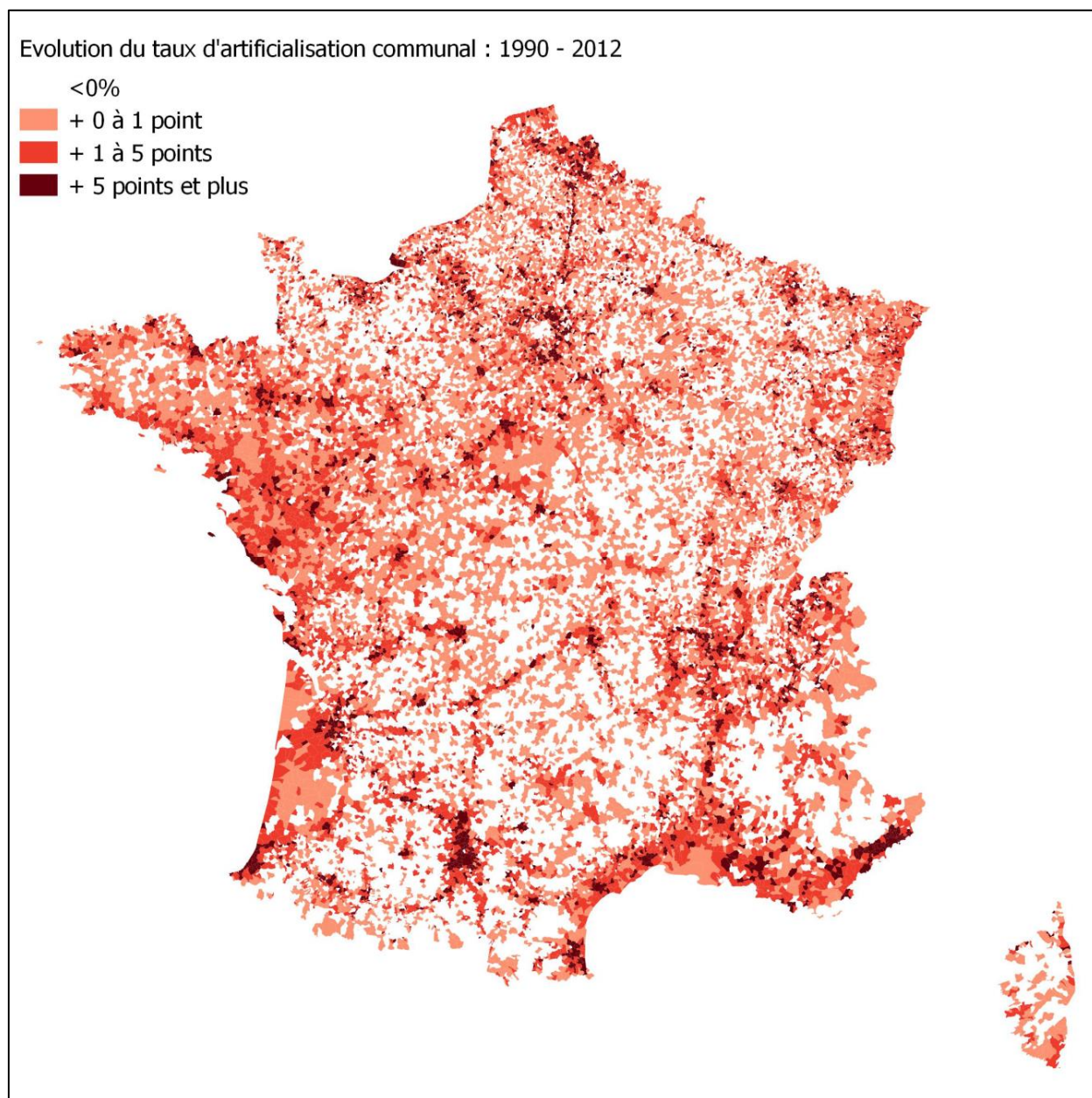
Figure 1 - Évolution des taux d'artificialisation communaux en France entre 1990 et 2012 (Source : Corine Land Cover 2012)
