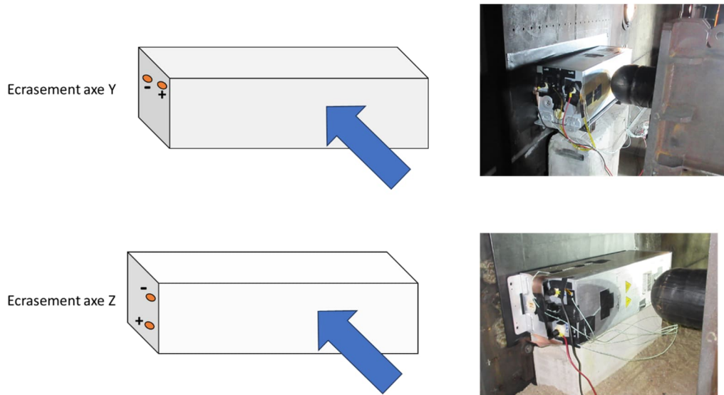
Figure 5 : Axes d'écrasement des modules
