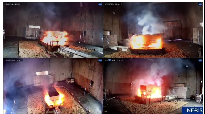
Photographie 30 : le feu gagne rapidement en intensité entretenu à l'intérieur de la caisse par la réaction du module.
