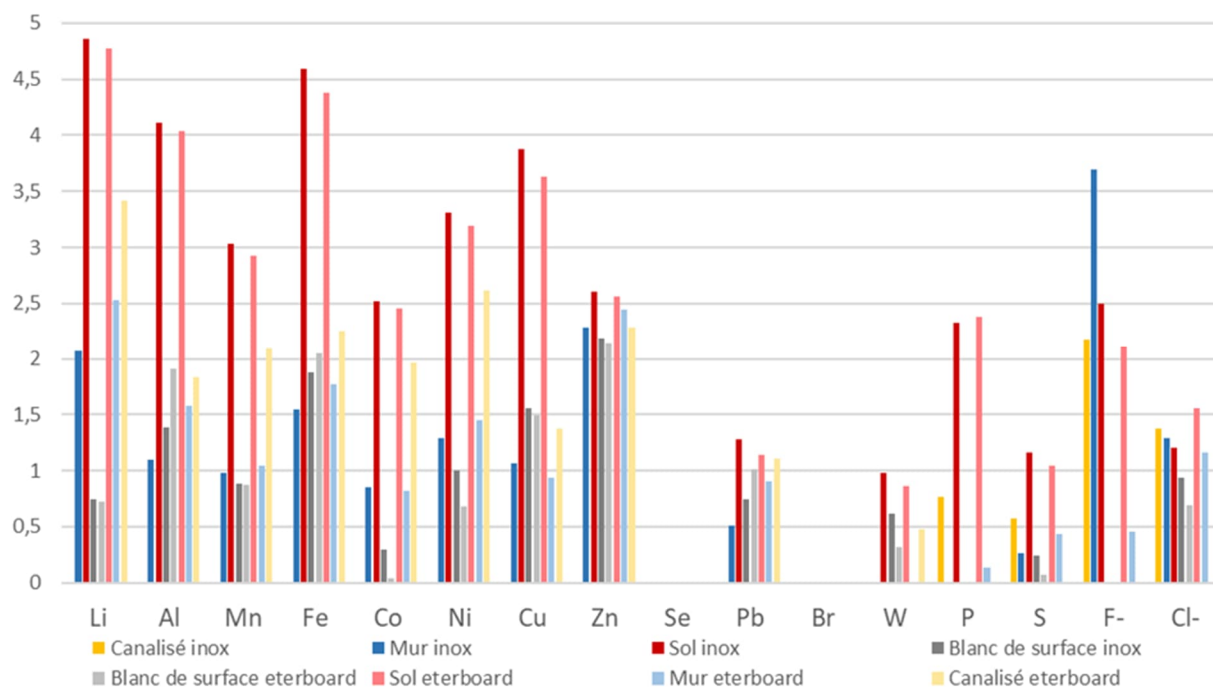
Figure 121 : Résultats des analyses élémentaires des prélèvements réalisés sur les supports placés dans la chambre lors de l'essai flux radiatif module
