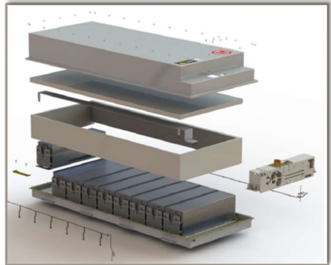
Figure 2 : Vue éclatée d'un pack batterie comprenant 9 modules et un BMS.
