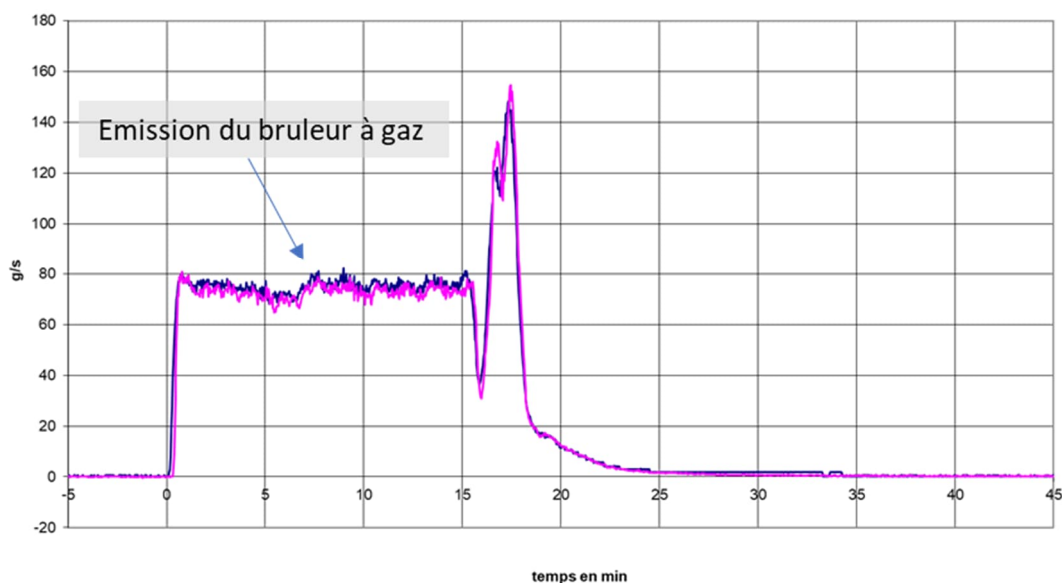
Figure 103 : Débit massique CO 2 essai de flux radiatif module
