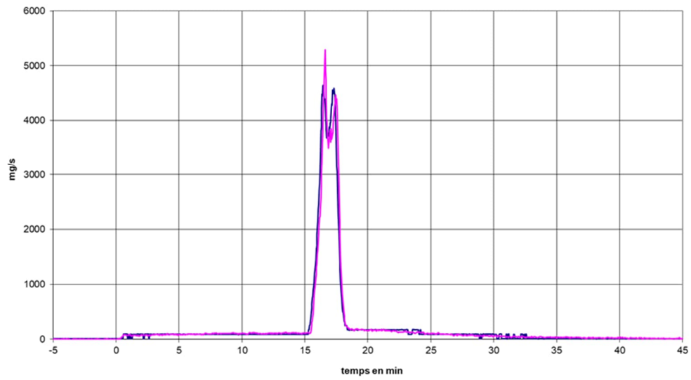
Figure 104 : Débit massique CO essai de flux radiatif module
