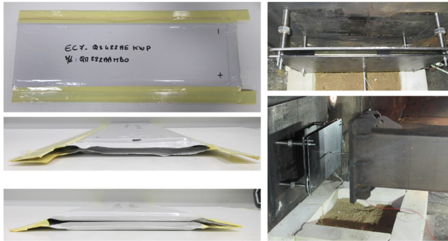
Figure 18 : Photographies de l'assemblage d'EC et du spécimen en position de test
