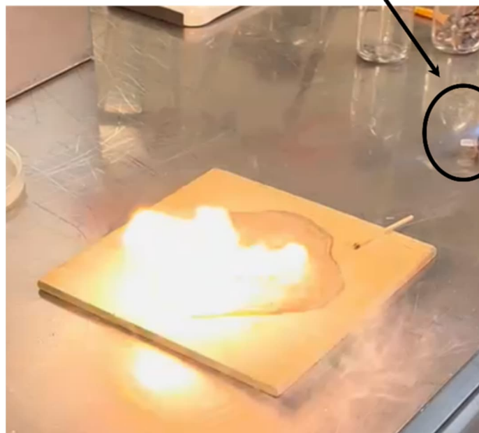
Figure 148 : Clichés photographiques de la tentative d'inflammation au brûleur à gaz des gaz générés lors de l'ajout de quelques gouttes d'eau sur l'échantillon soumis à la phase 3 de l'épreuve N.5
