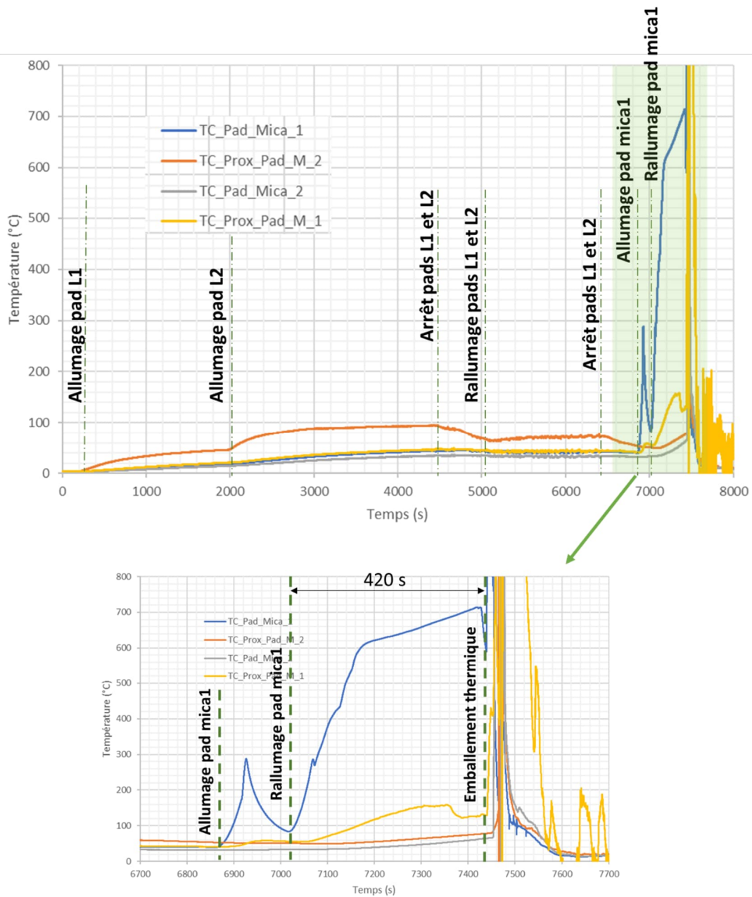
Figure 30 : Températures mesurées par les thermocouples sur et à proximité des éléments chauffants en mica
