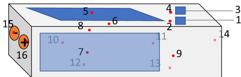
Figure 26 : Positionnement des thermocouples pour l'essai de chauffe localisée
