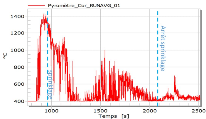
Figure 87 : Température maximale (sur un pixel) enregistrée par la caméra thermique (haut) et température enregistrée par le pyromètre (bas). Les mesures de températures durant le sprinklage peuvent être affectées par la présence de gouttelettes d'eau entre le feu et l'objectif de la caméra.
