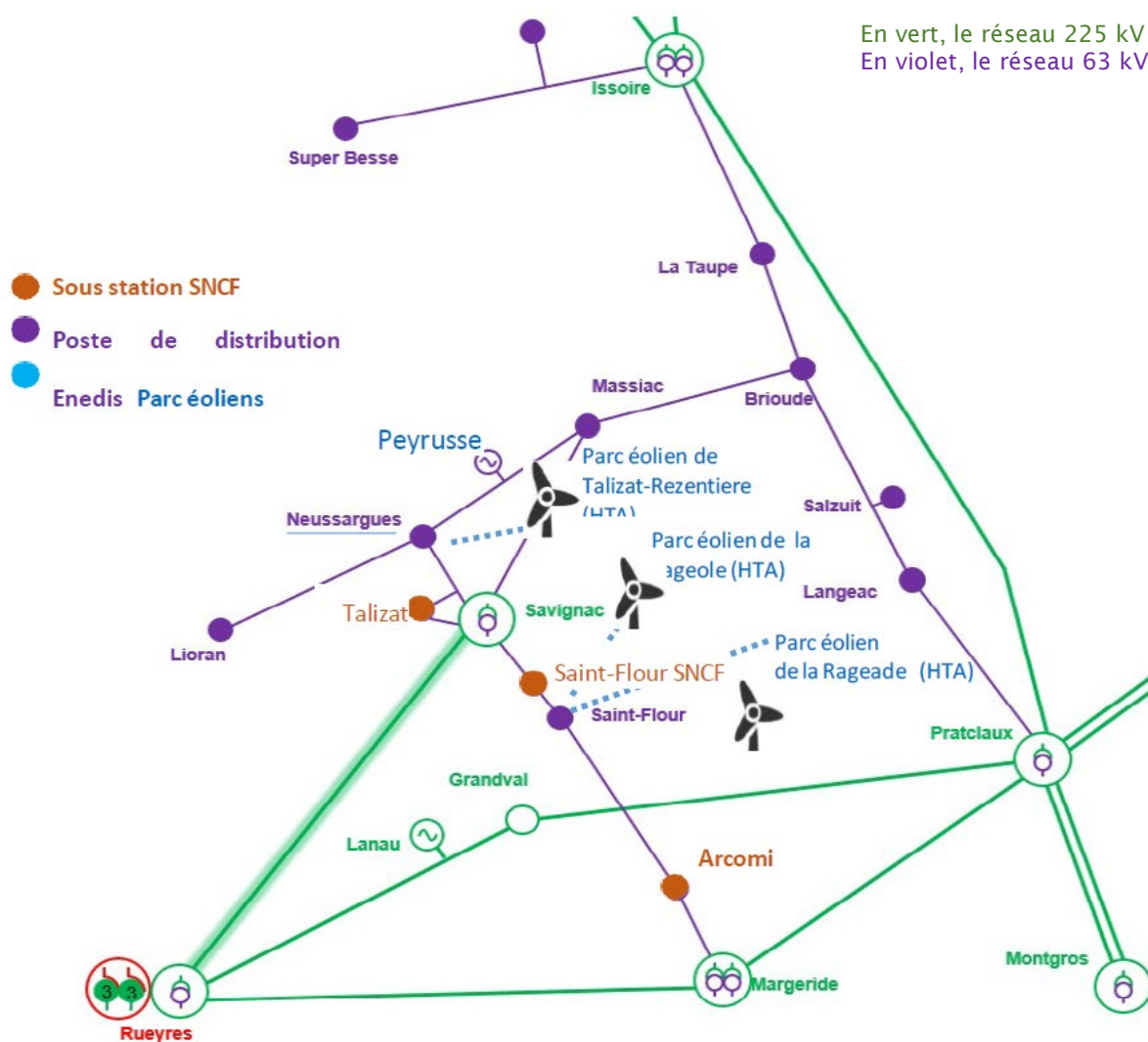
Figure 1 : Schéma électrique de la zone (source : dossier)
