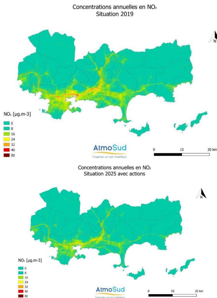
Figure 4 : Cartes modélisées de la pollution de l'air aux oxydes d'azote en 2019 et en projection à l'horizon 2025 avec mesures du PPA. Source : étude d'AtmoSud
