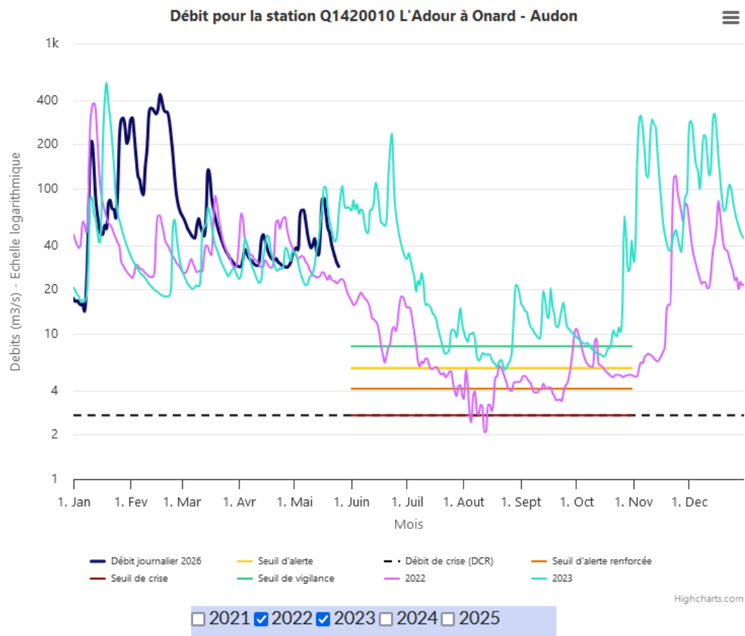
Figure 13 Exemple d'évolution de débit et comparaison interannuelle
