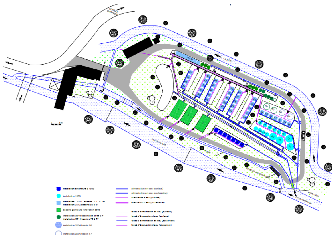
Plan de la pisciculture de Pont-Crouzet Source : MIGADO
