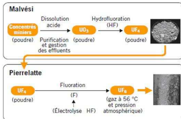
Figure 2 : Principales étapes du procédé de conversion de COMURHEX
