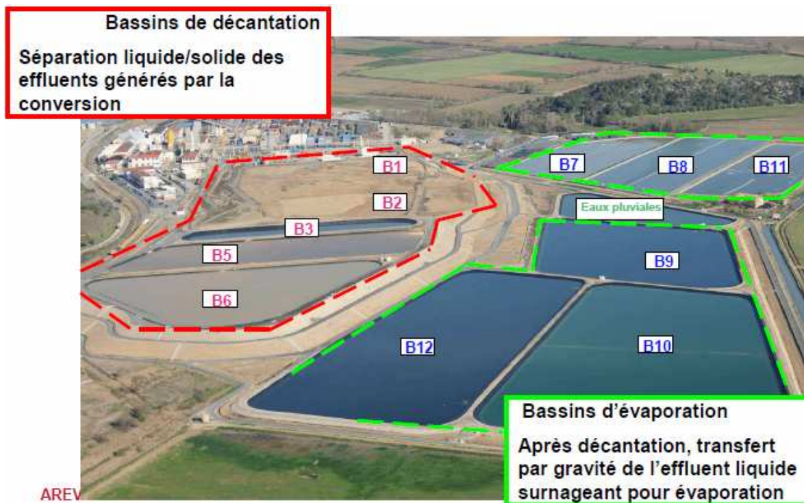
Figure 3 : Les différents bassins de l'Etablissement COMURHEX de Malvézi (photo prise en direction du nord, document transmis aux rapporteurs par le maître d'ouvrage).
